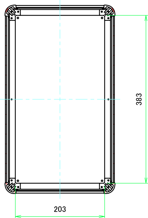
B-B ( 1:5 )
