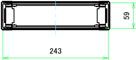
C-C ( 1:5 )
