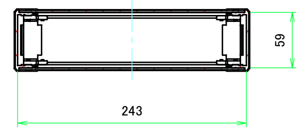
C-C ( 1:4 )
