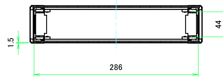
A-A ( 1:4 )
