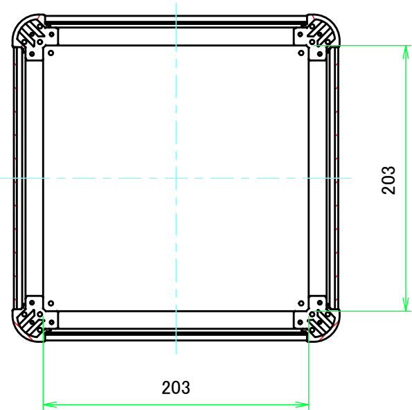
B-B ( 1:4 )
