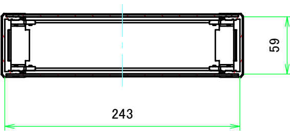
C-C ( 1:4 )
