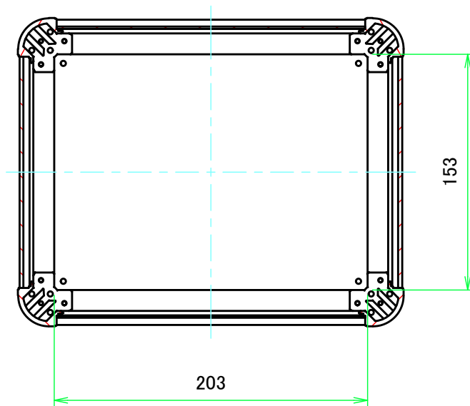
B-B ( 1:3.5 )
