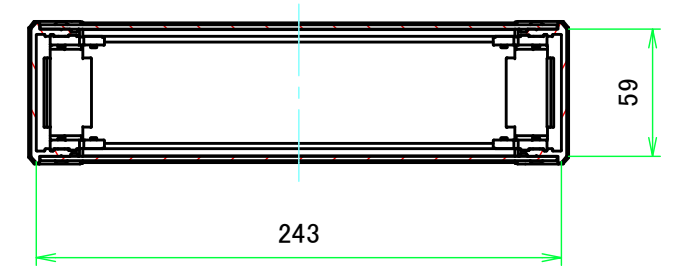
C-C ( 1:3.5 )
