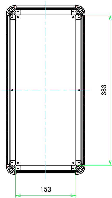
B-B ( 1:5 )
