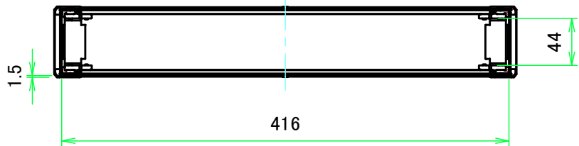
A-A ( 1:5 )
