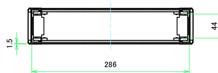
A-A ( 1:4 )
