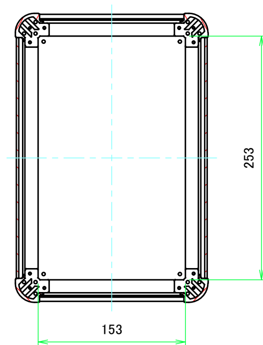
B-B ( 1:4 )
