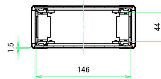
A-A ( 1:3.5 )
