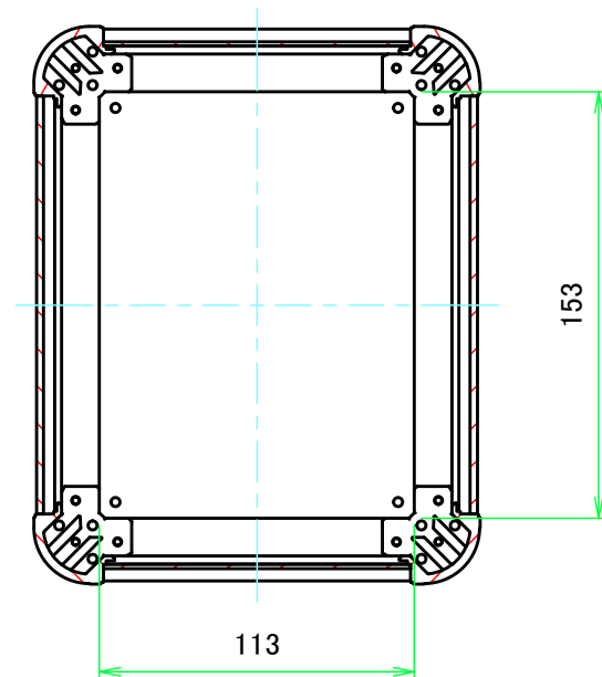
B-B ( 1:3 )
