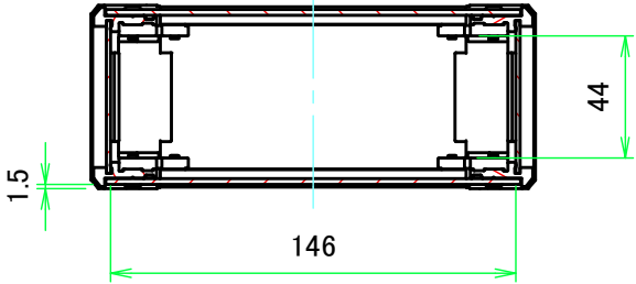
A-A ( 1:3 )
