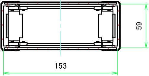
C-C ( 1:3 )
