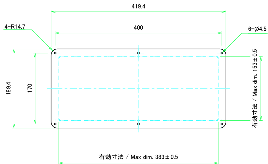
保護シート側 Surface protective film side
