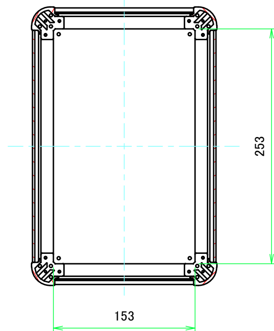
B-B ( 1 : 4 )
