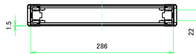
A-A ( 1 : 4 )
