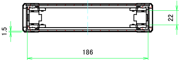
A-A ( 1 : 3 )
