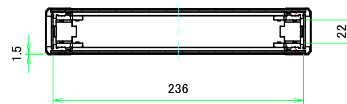
A-A ( 1 : 3.5 )
