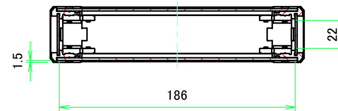
A-A (1:3)
