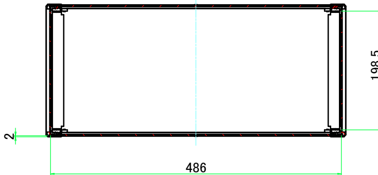
A-A ( 1 : 6.5 )
