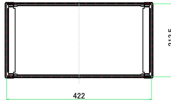
C-C ( 1 : 6.5 )
