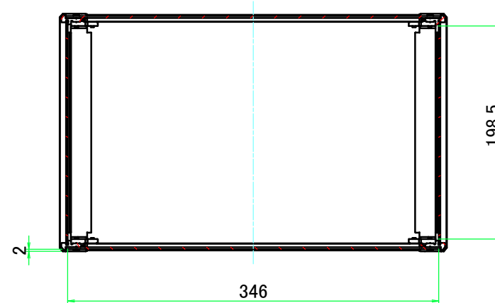
A-A (1:5)
