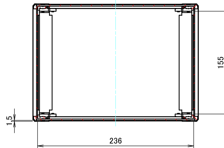
A-A ( 1 :3.5 )
