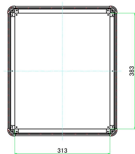
B-B ( 1 : 6 )
