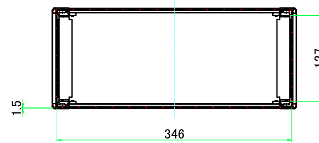
A-A ( 1 : 5.5 )
