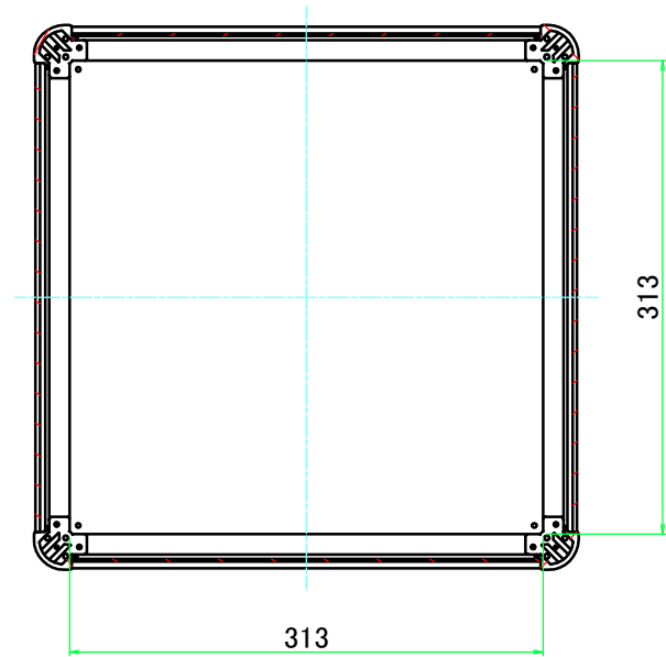
B-B ( 1 : 5.5 )
