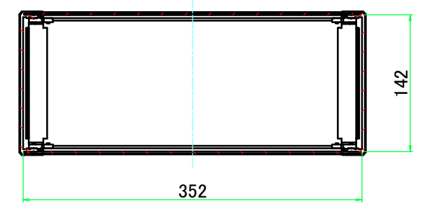
C-C ( 1 : 5.5 )
