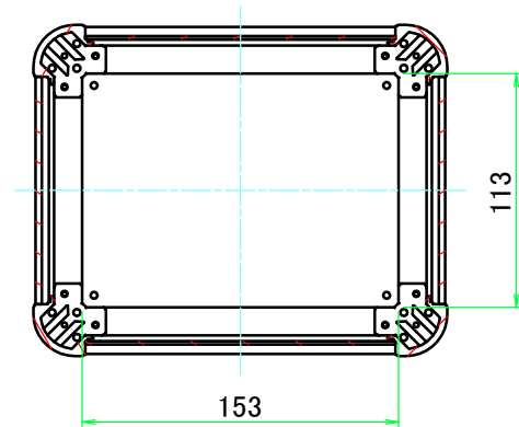
B-B ( 1 : 4 )
