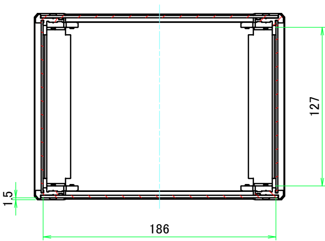
A-A ( 1 : 3 )
