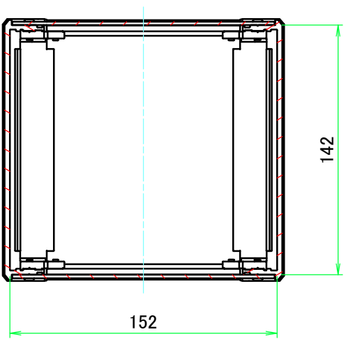
C-C ( 1 : 3 )
