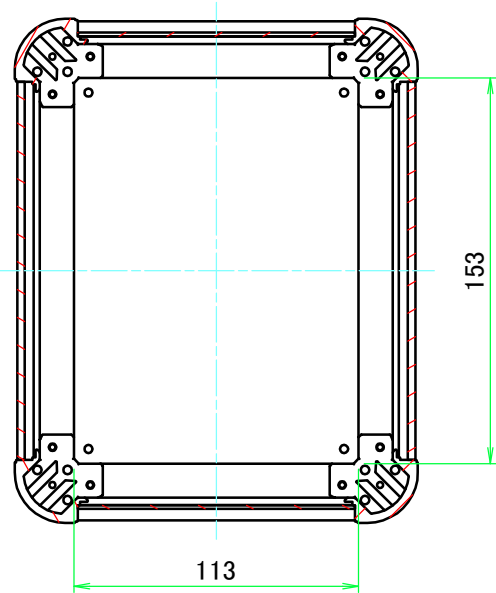
B-B ( 1 : 3 )
