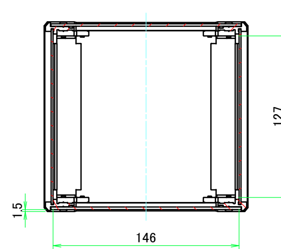
A-A (1:3)
