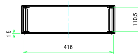
A-A (1:7.5)
