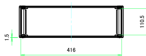
A-A (1:6.5)
