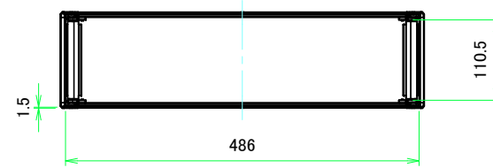
A-A (1:6.5)
