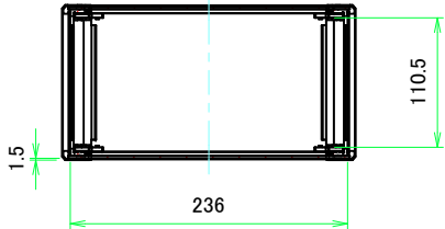
A-A (1:5)
