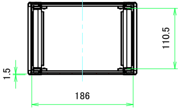
A-A (1:5)
