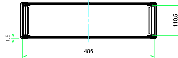
A-A (1:6)
