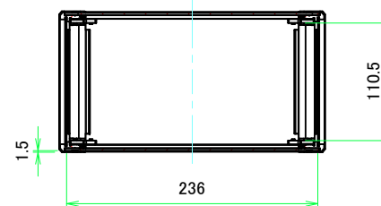
A-A (1:4.5)
