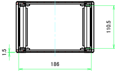
A-A (1:4)
