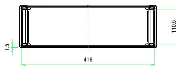
A-A (1:5)
