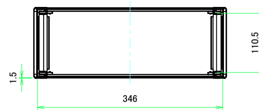
A-A (1:5)
