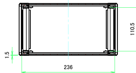
A-A (1:4)
