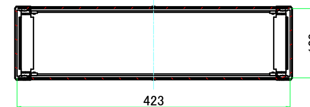
C-C ( 1 : 6 )
