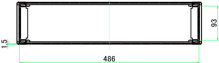
A-A ( 1 : 6 )
