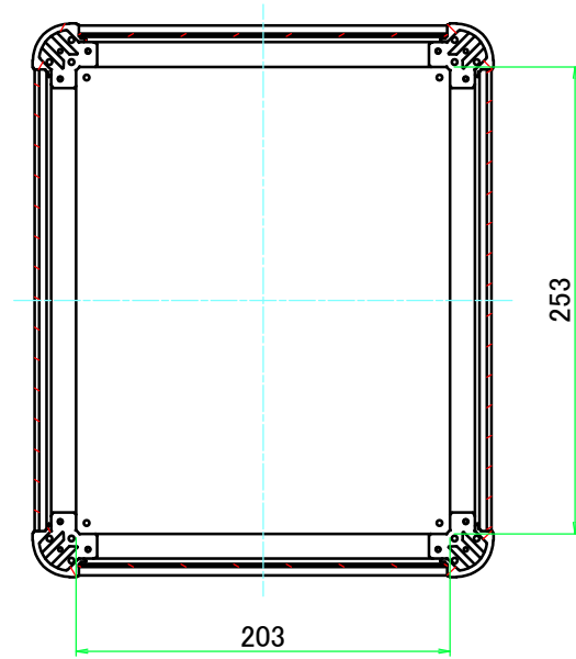
B-B ( 1 : 4.5 )
