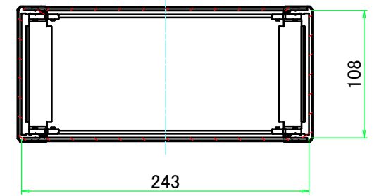
C-C ( 1 : 4.5 )
