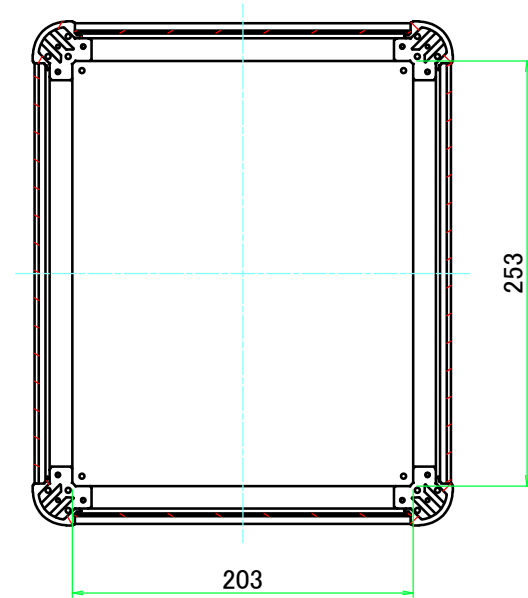
B-B ( 1 : 4.5 )
