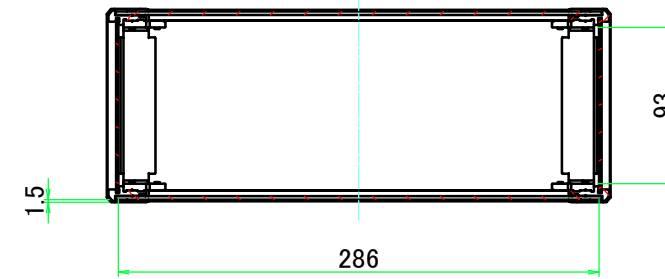
A-A ( 1 : 4.5 )
