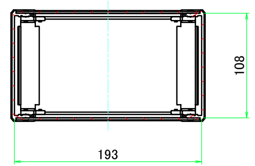
C-C ( 1 : 4 )
