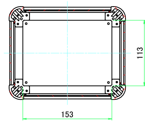
B-B ( 1 : 4 )
