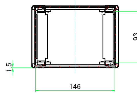
A-A ( 1 : 4 )
