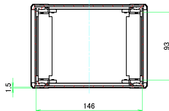
A-A ( 1 : 3 )
