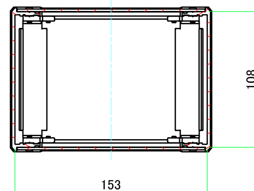
C-C ( 1 : 3 )
