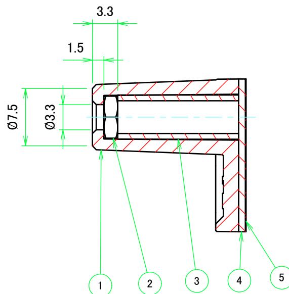
A-A (2:1)
