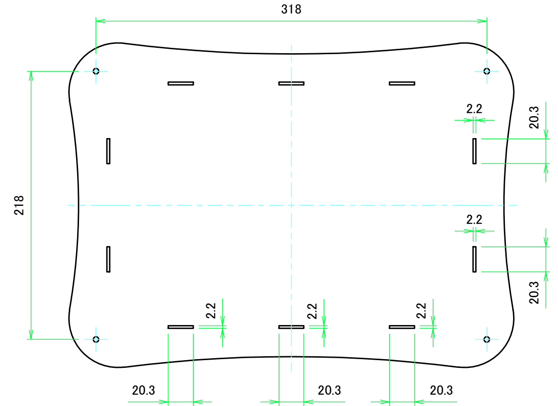
上カバー裏面 / Top cover Backside
