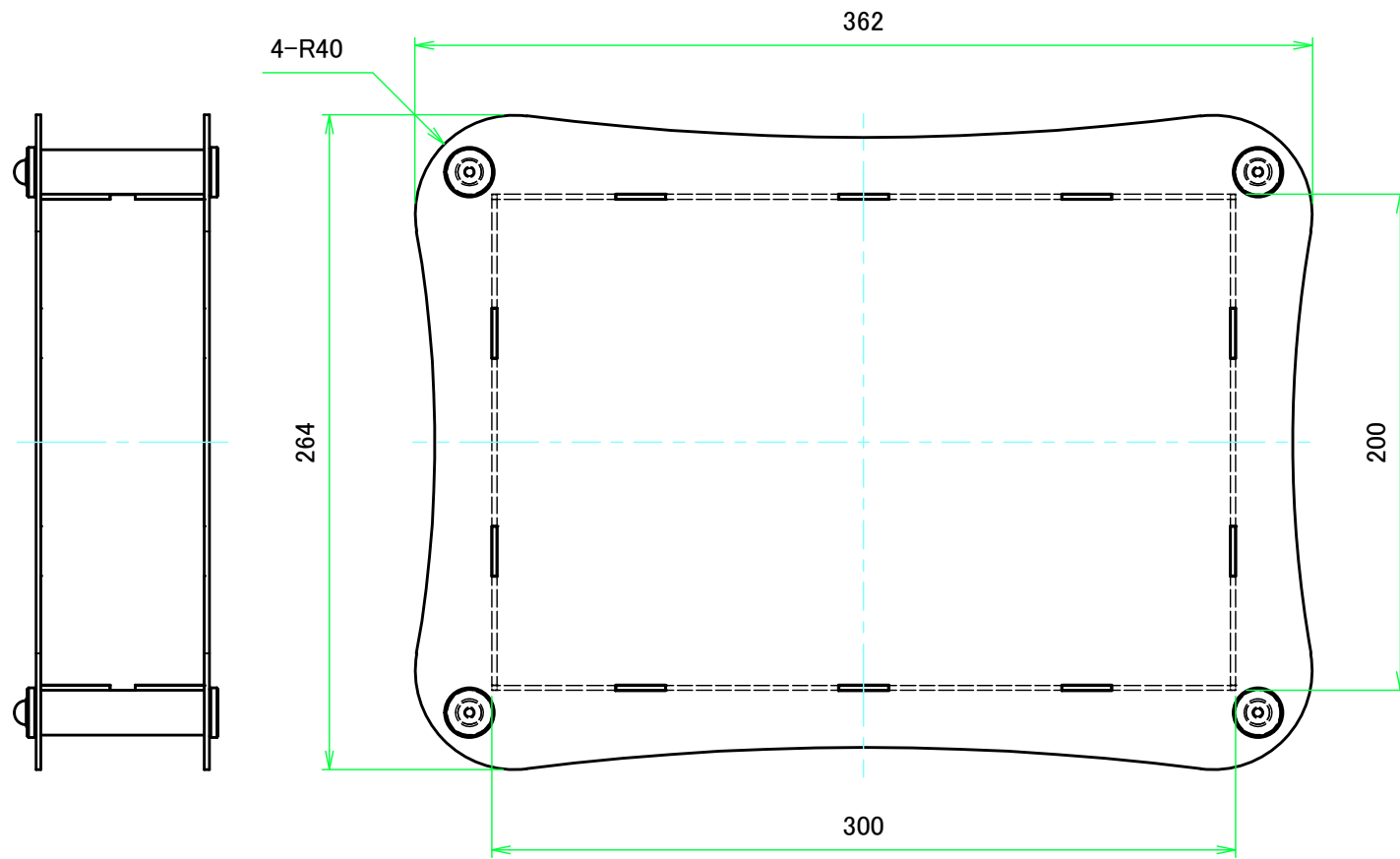
Dパネル2 / D Panel 2
