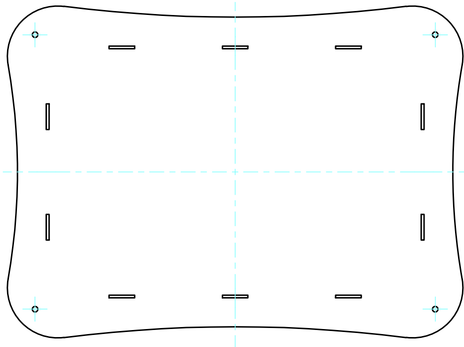
下カバー表面 / Bottom cover Frontside
