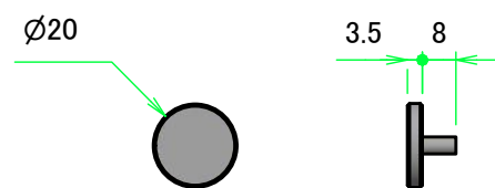
取付用ローレットビス / Knurled Thumb Screw
