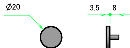
取付用ローレットビス / Knurled Thumb Screw
