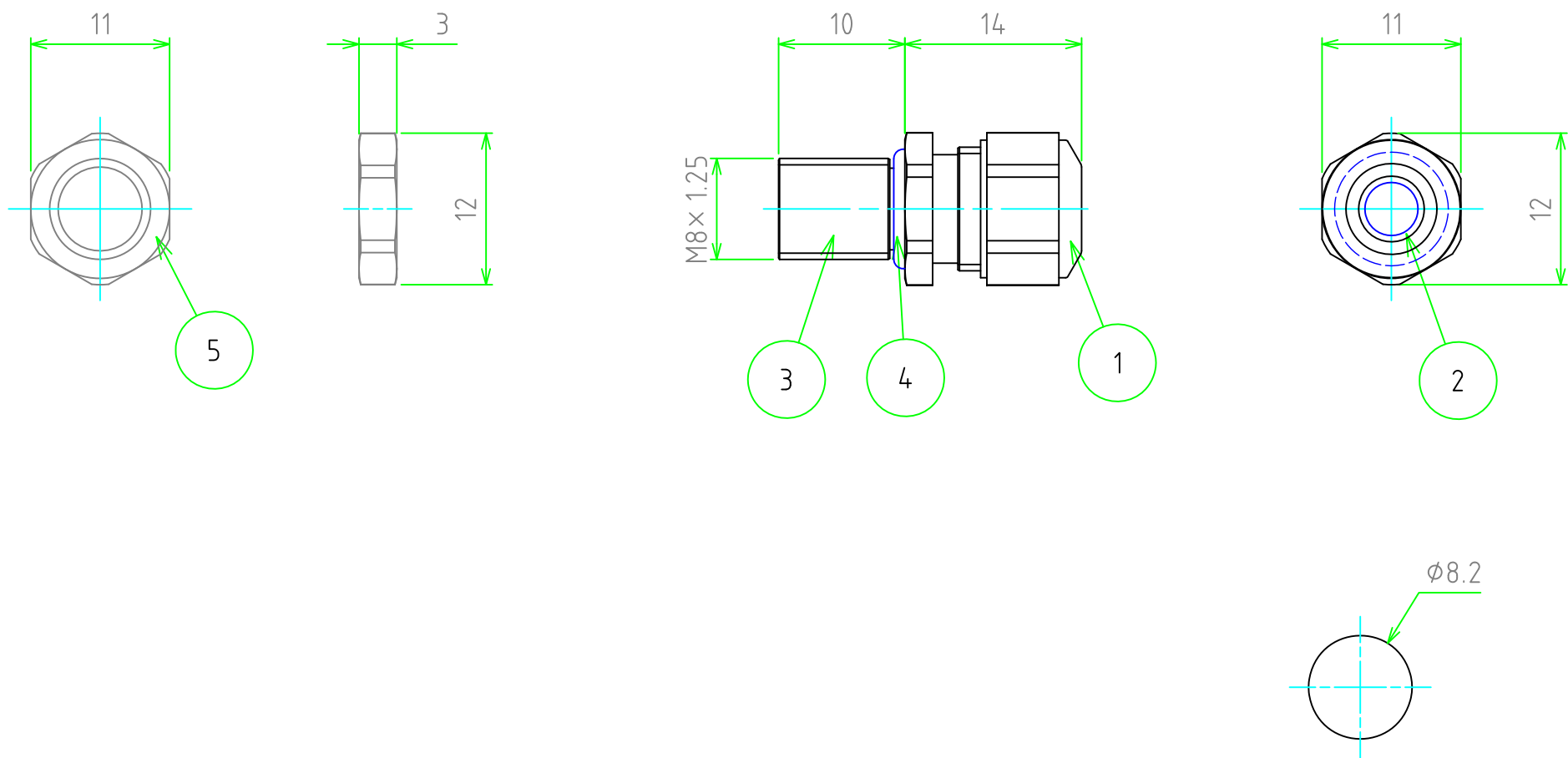
取付穴寸法 / Mounting hole dimensions
