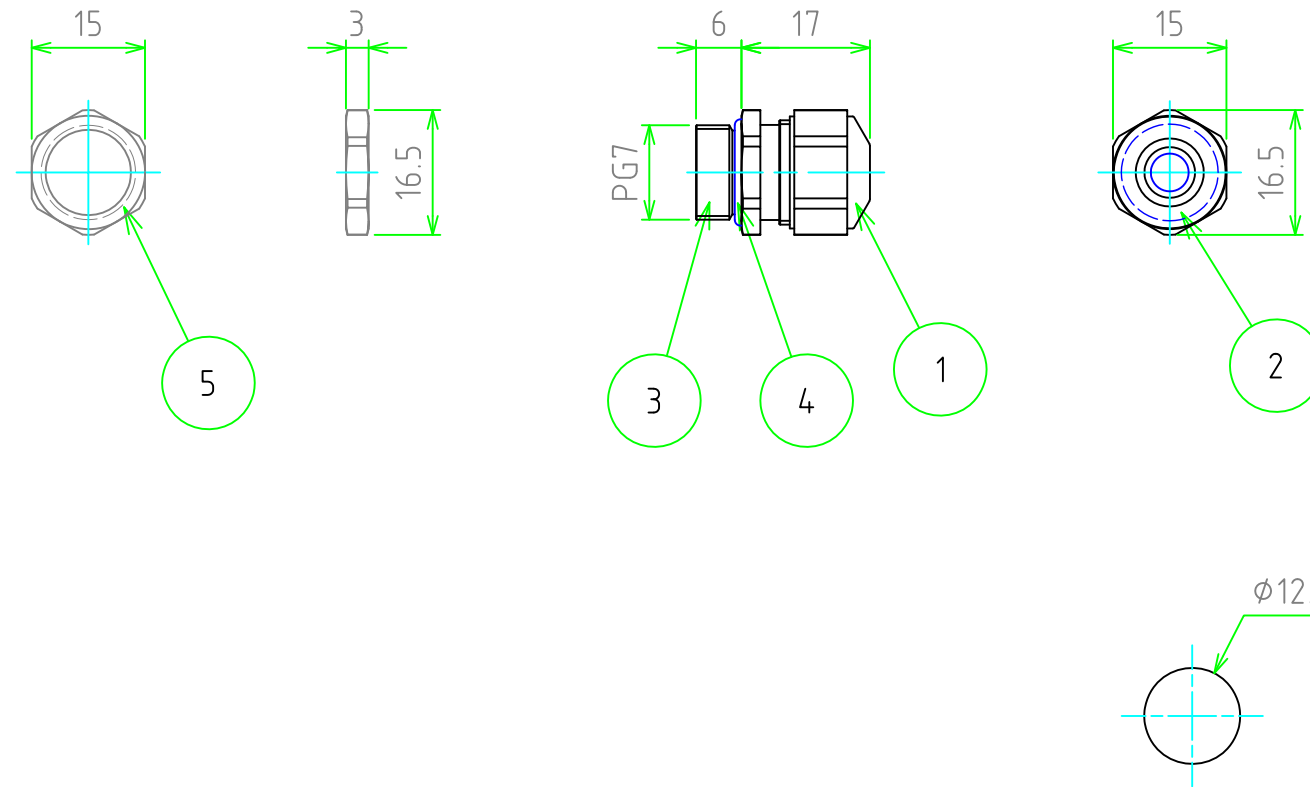
取付穴寸法 / Mounting hole dimensions
