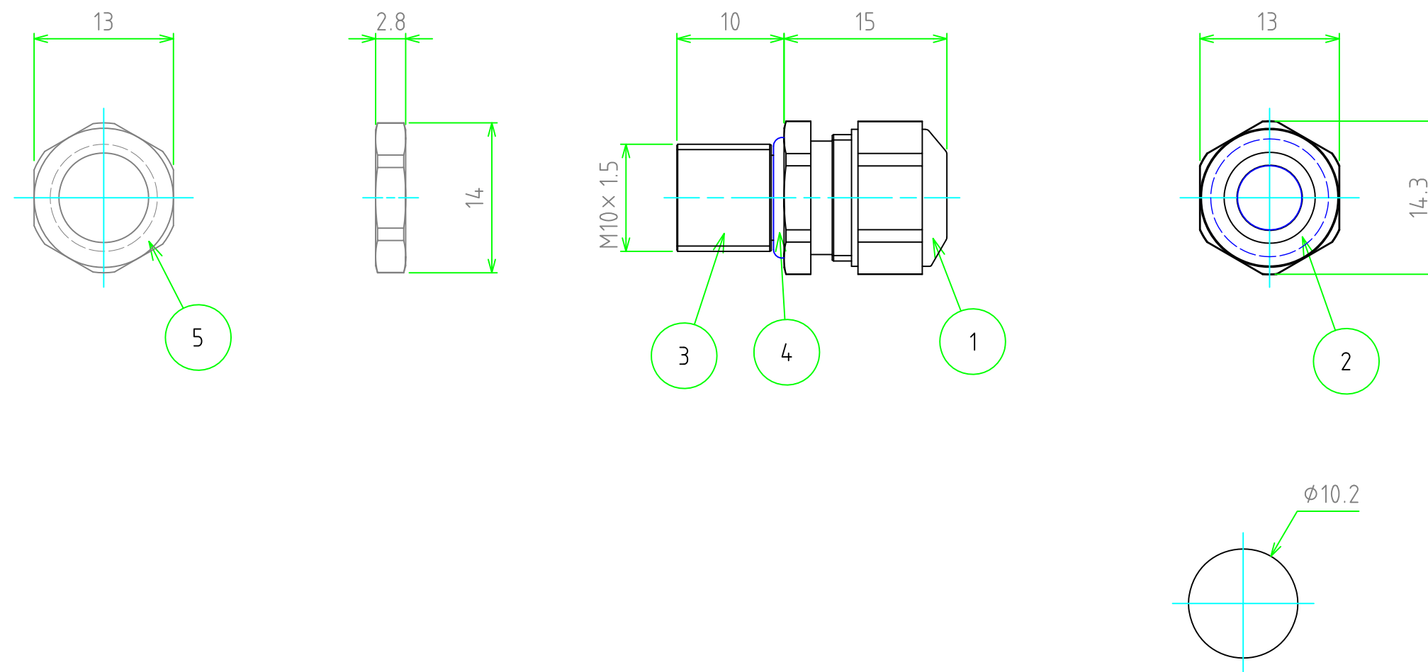
取付穴寸法 / Mounting hole dimensions
