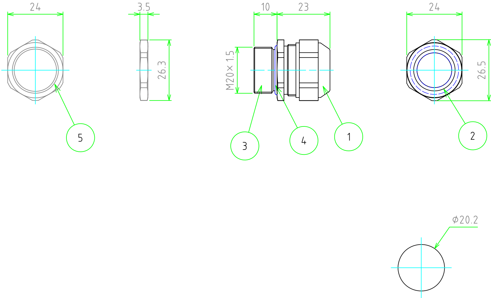
取付穴寸法 / Mounting hole dimensions
