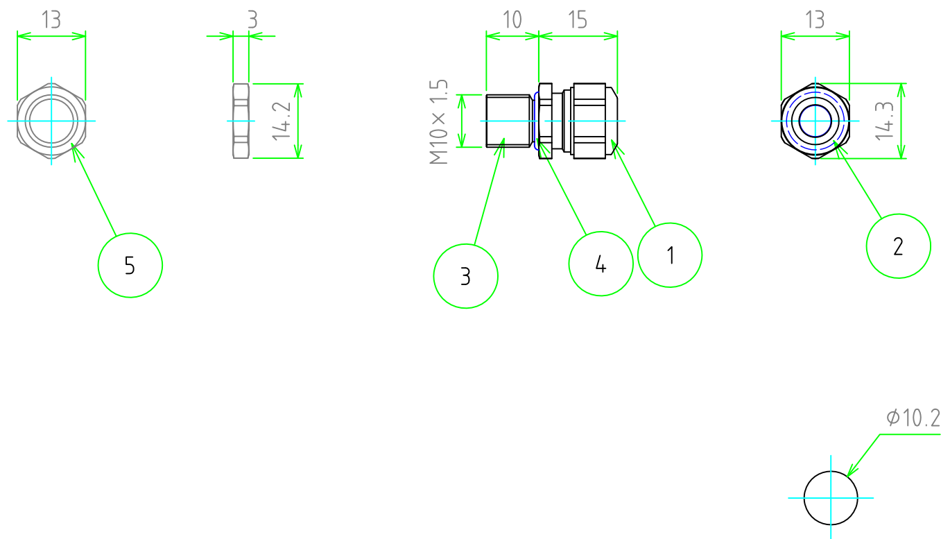
取付穴寸法 / Mounting hole dimensions
